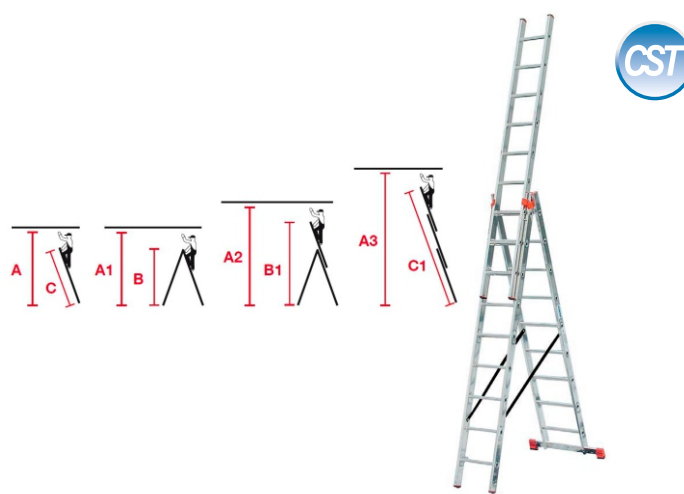
Scară KRAUSE multifuncțională din aluminiu - 3 tronsoane -
