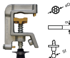
UNIVERSAL CLASSIC REDUCED CLAMP (CCRU/B)
